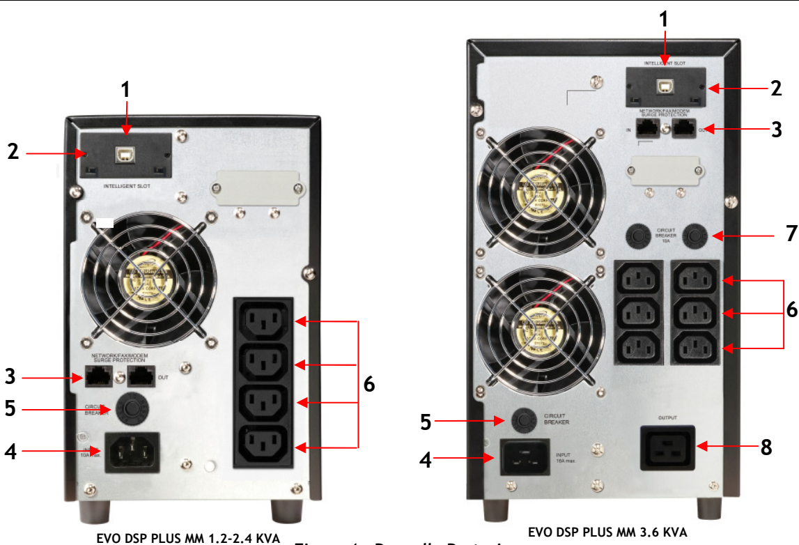
Figura 4 - Pannello Posteriore
